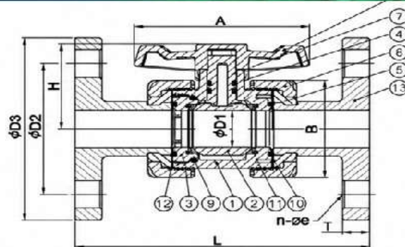
15A-50A FLANGE TYPE
